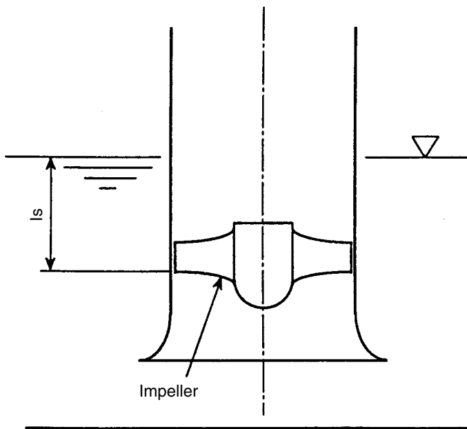
Fig. 1-5 NPSH av.
